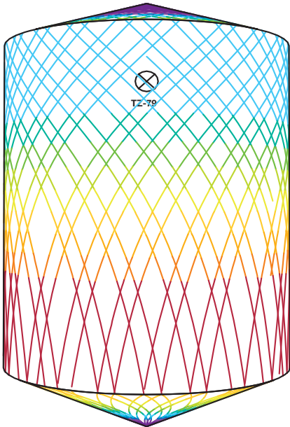
D8m H10m, Toftejorg TZ-79, 4 x ø10 mm, 0 % 时间 = 5.5 分钟, 耗水量 = 2565 升
