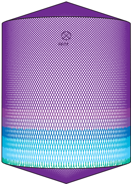
D5m H6m, Toftejorg TZ-74自清洁型4 x ø7 mm, 0%时间 = 15。3分钟，耗水量 = 4853 l
