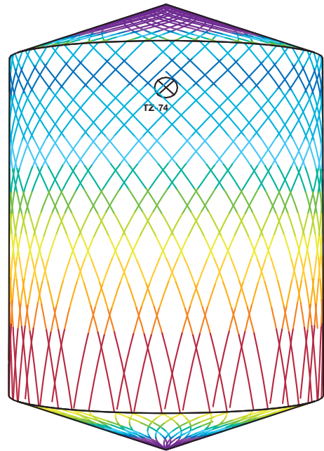
D5m H6m, Toftejorg TZ-74自清洁型4 x ø7 mm, 0%时间 = 3。8分钟，耗水量 = 1192 l
