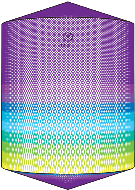
D2.5m H6m, Toftejorg TZ-67, 4 x ø6 mm 时间 = 14.7 分钟，耗水量 = 3097 升
