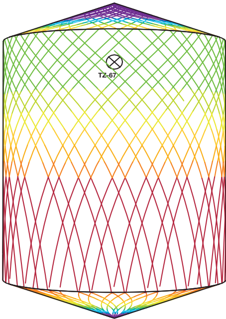
D2.5m H6m, Toftejorg TZ-67, 4 x ø6 mm 时间 = 3.5 分钟，耗水量 = 727 升
