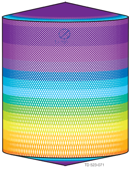
D4. 6m H5.5m, Toftejorg MultiJet 25. 4 x ø5.5 mm, 时间 = 8.3 分钟, 耗水量 = 1612 升
