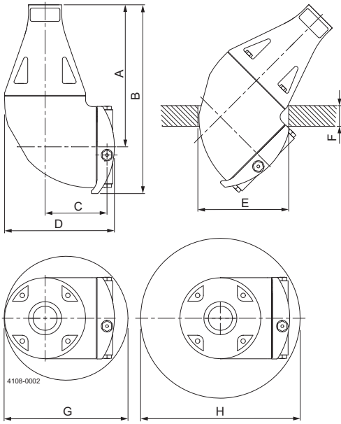
尺寸 (mm)
