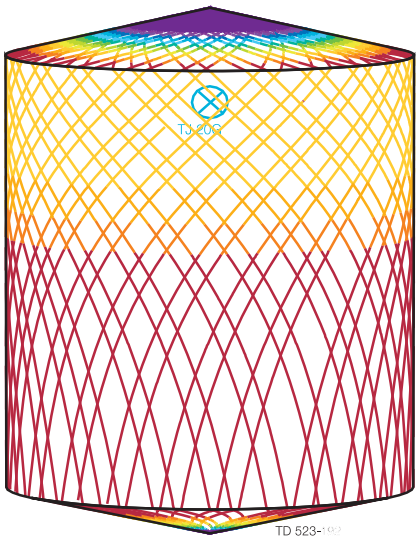
D4. 6m H5.5m, Toftejorg MultiJet 25. 4 x ø5.5 mm, 时间 = 2.08 分钟, 耗水量 = 403 升
